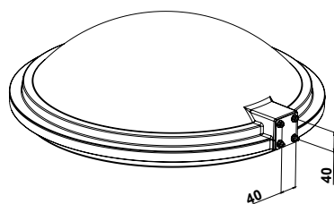
BEZPOŚREDNI Kwadratowy (C40x40)
