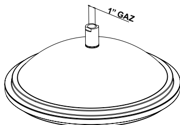
BEZPOŚREDNI Żeński uchwyt montażowy 1" (G34F)
